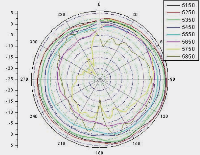
5G (PHI=90)
