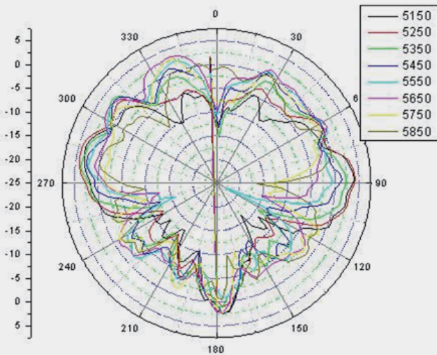
5G (PHI=0)
